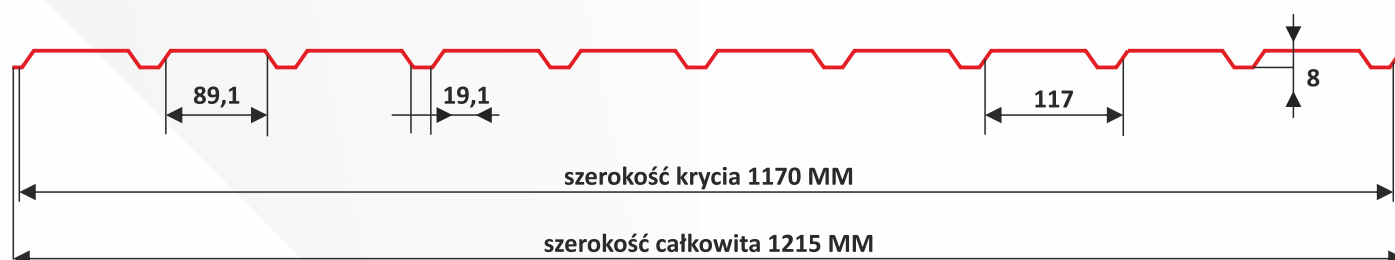
PROFIL DACHOWY D / PROFIL ELEWACYJNY E
