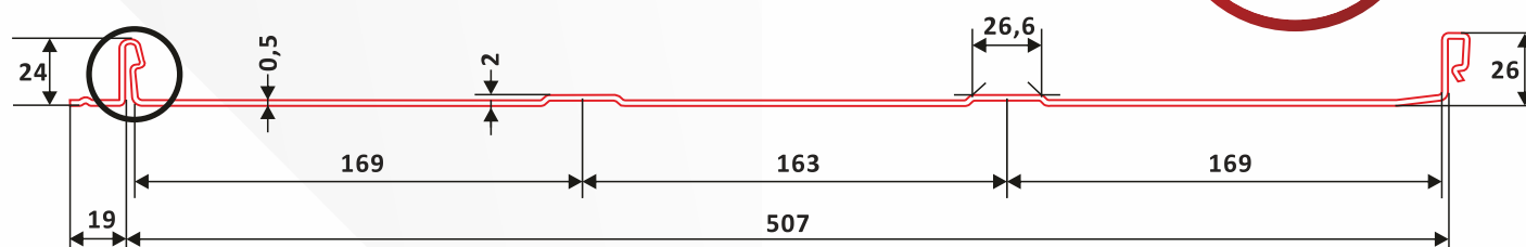
PRZEKRÓJ BLACHY TRAPEZOWEJ
